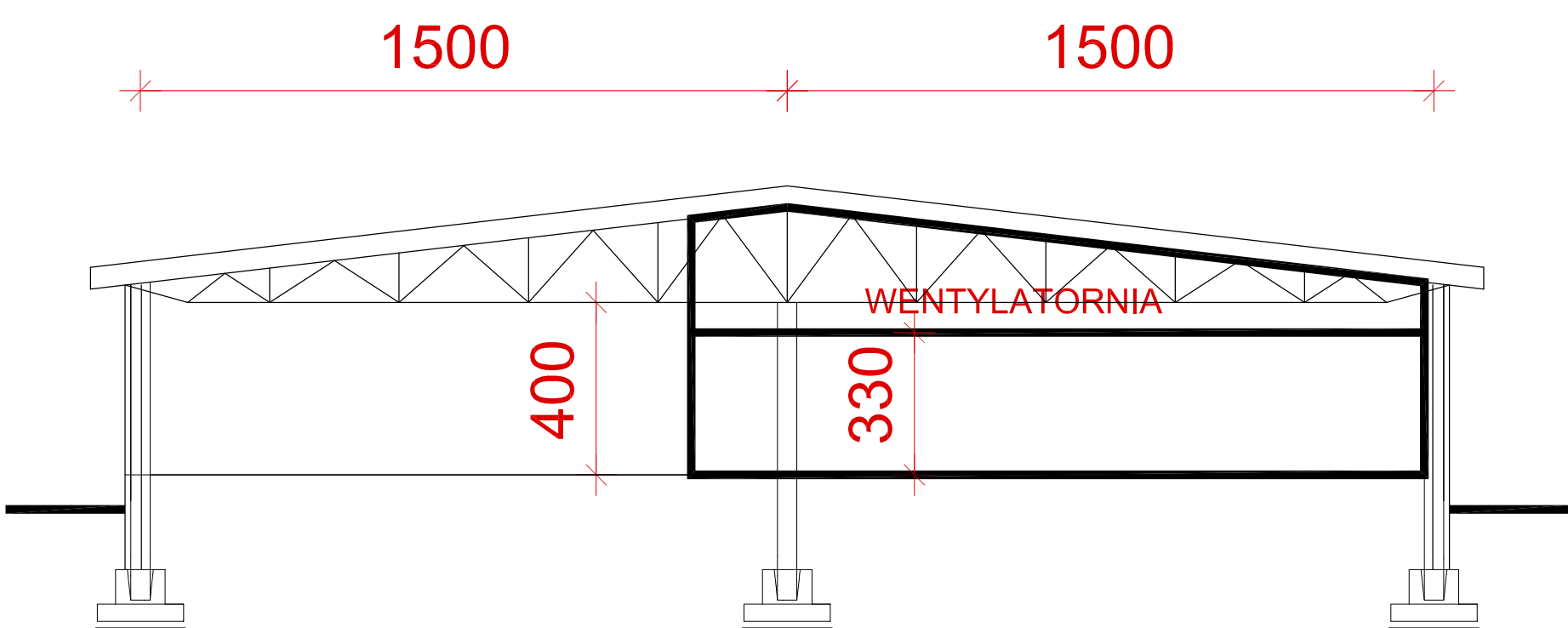
PRZEKRÓJ III-III
