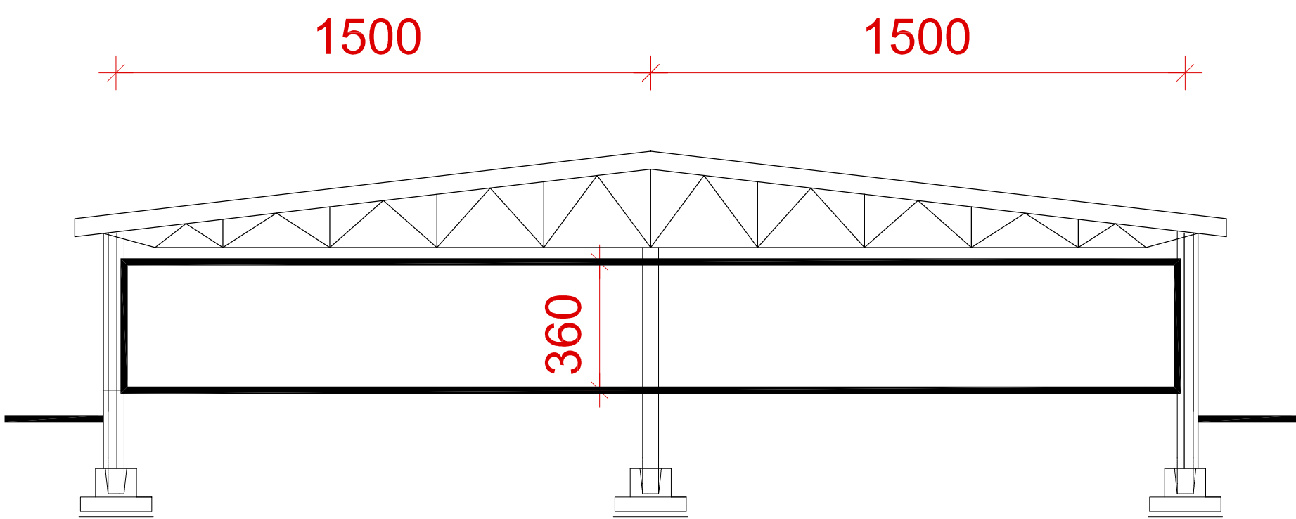
PRZEKRÓJ I-I
