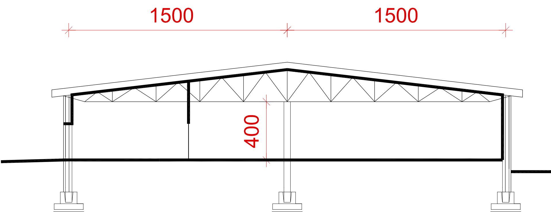
PRZEKRÓJ II-II
