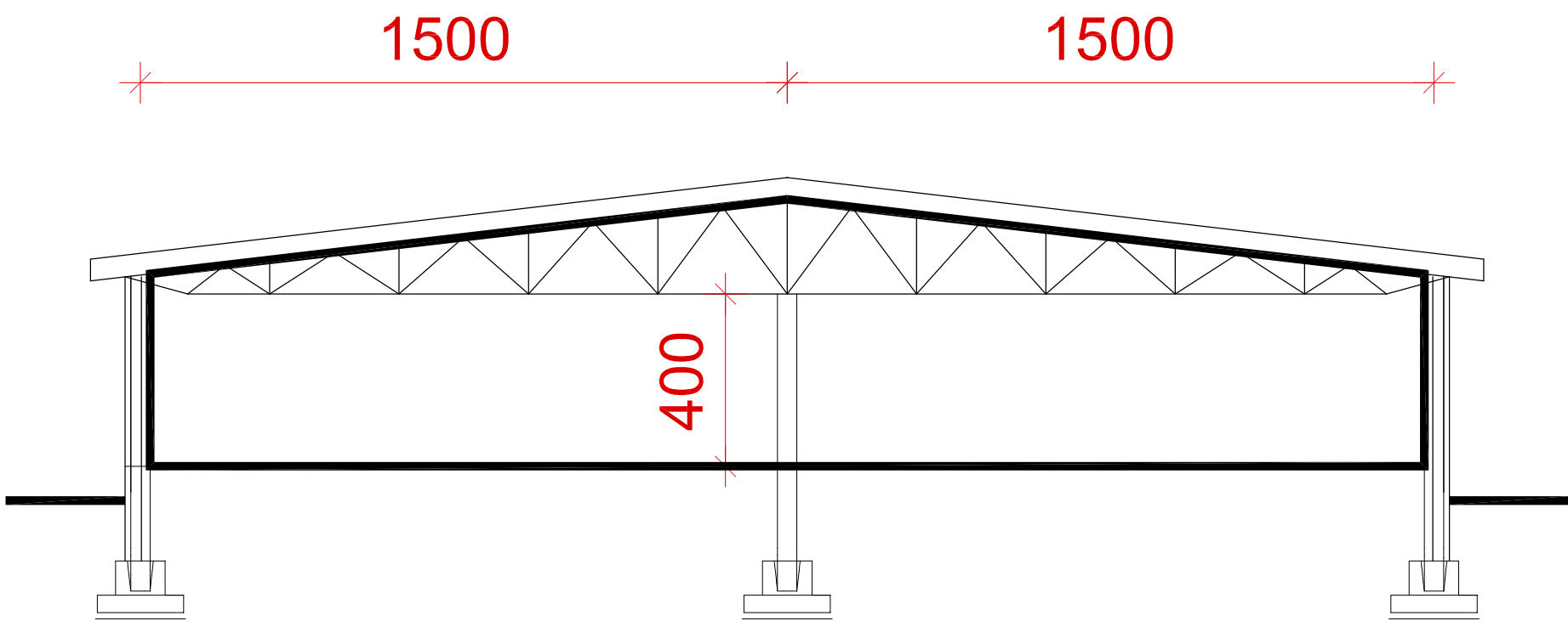
PRZEKRÓJ IV-IV
